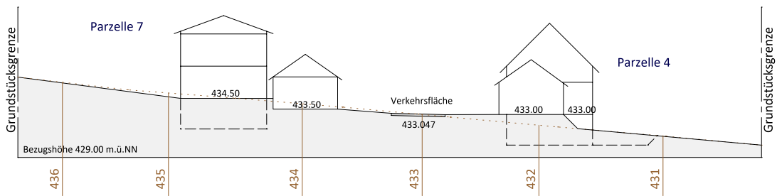
Schnitt D-D M 1:500
