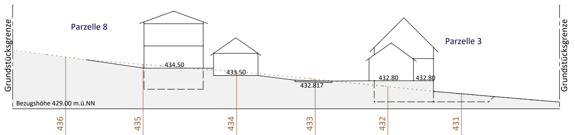
Schnitt C-C M 1:500
