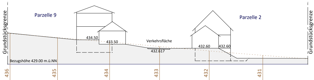
Schnitt B-B M 1:500
